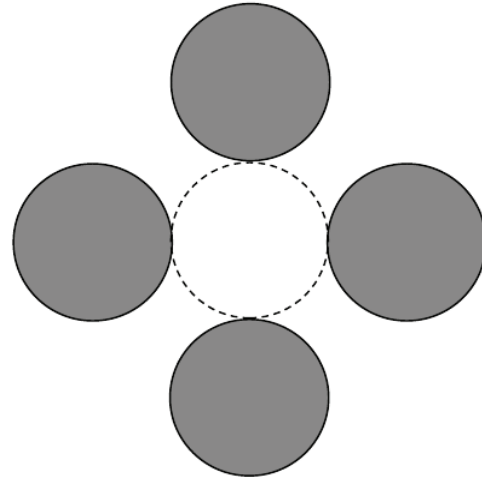
Quadrupole (n=2)
